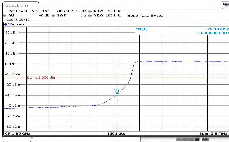
Band2-3MHz-QPSK-18615-15RB#0
