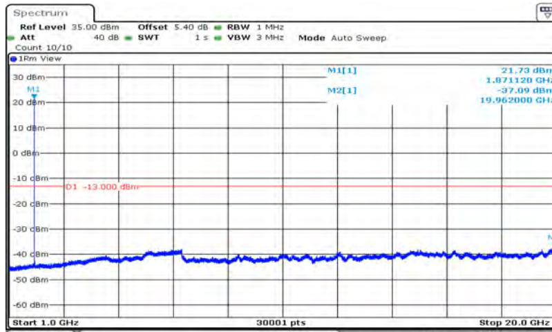
Band2-20MHz-64QAM-18900-1RB#0-Range2:1000~20000MHz
