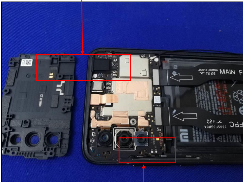
BT/WIFI/GPS Antenna
