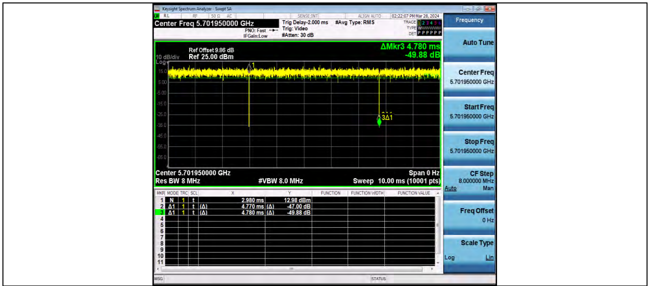
11AX20MIMO_Ant2_5700_26Tone_RU8
