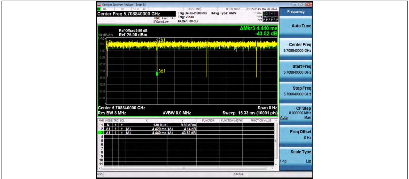
11AX20MIMO_Ant1_5700_52Tone_RU40
