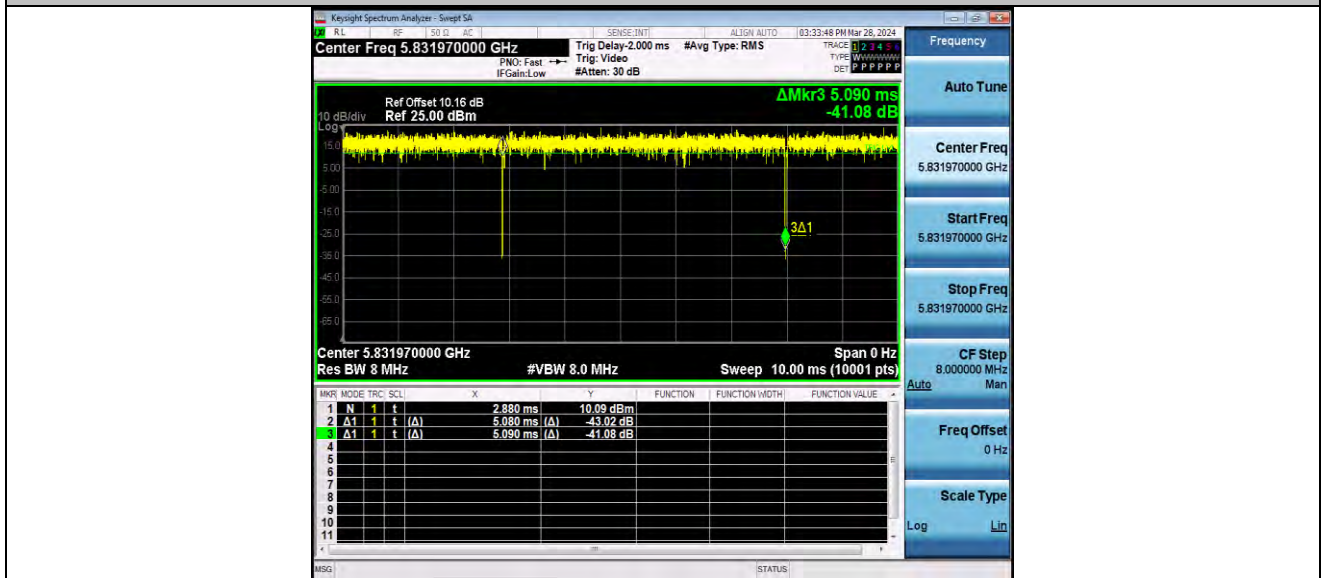
11AX20MIMO_Ant1_5825_106Tone_RU54
