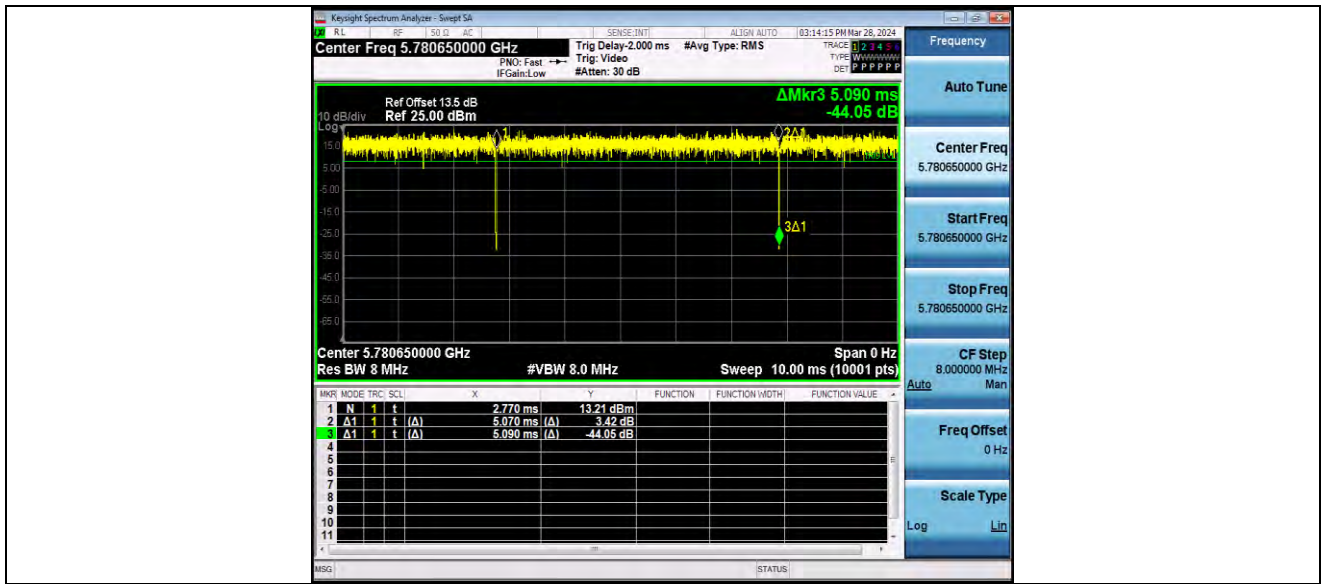
11AX20MIMO_Ant2_5785_106Tone_RU53
