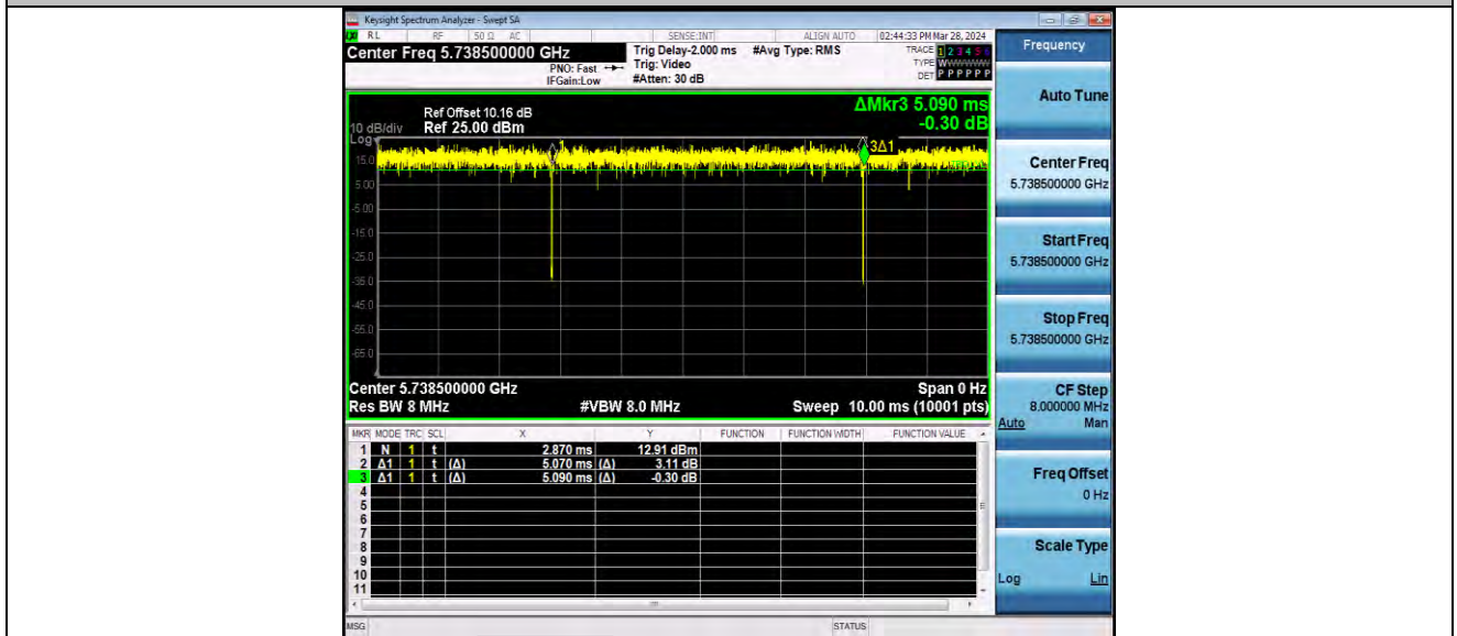
11AX20MIMO_Ant1_5745_106Tone_RU53
