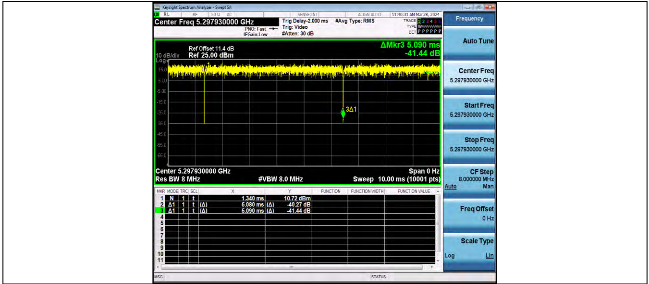
11AX20MIMO_Ant2_5300_106Tone_RU53
