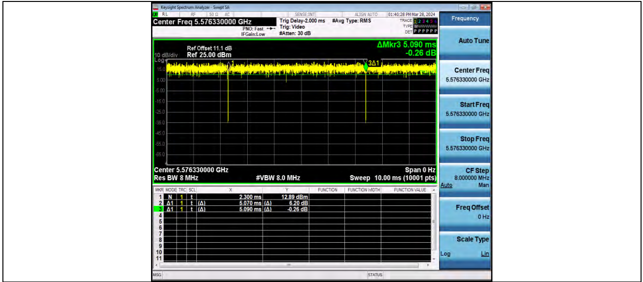
11AX20MIMO_Ant2_5580_106Tone_RU53
