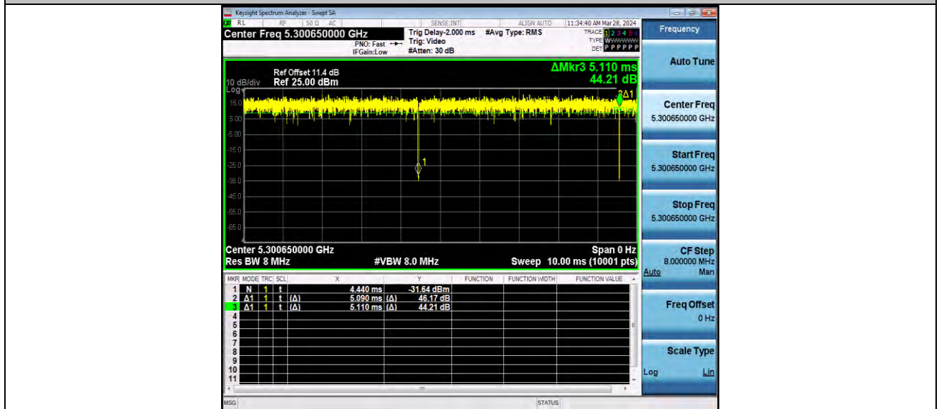
11AX20MIMO_Ant2_5300_52Tone_RU38
