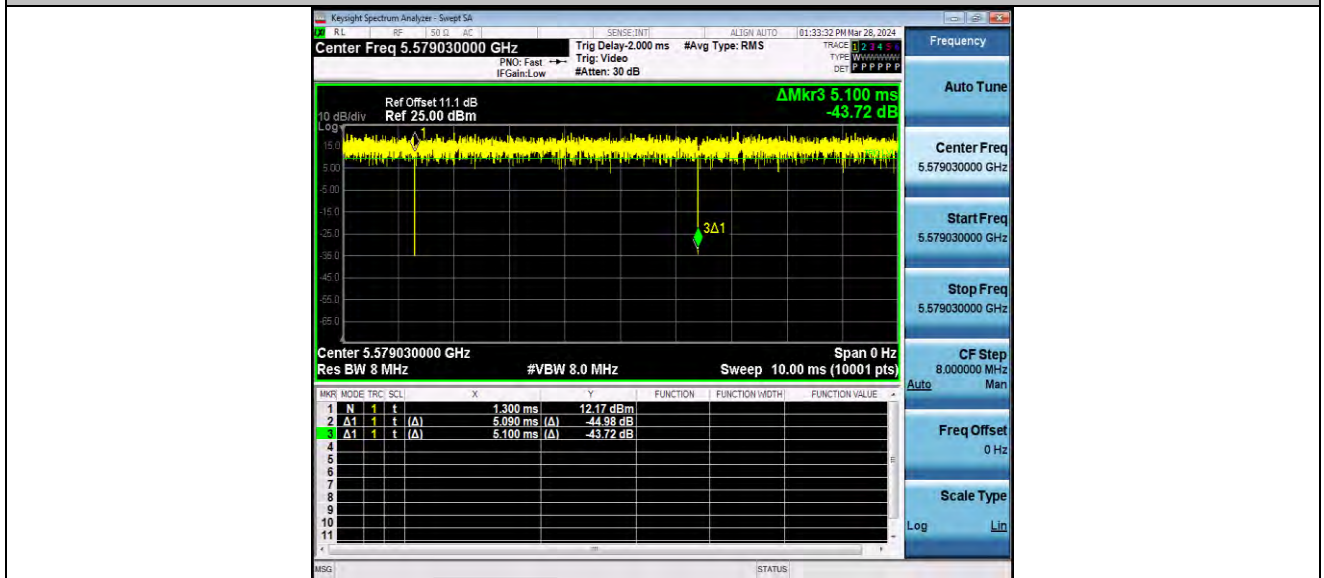
11AX20MIMO_Ant2_5580_52Tone_RU38
