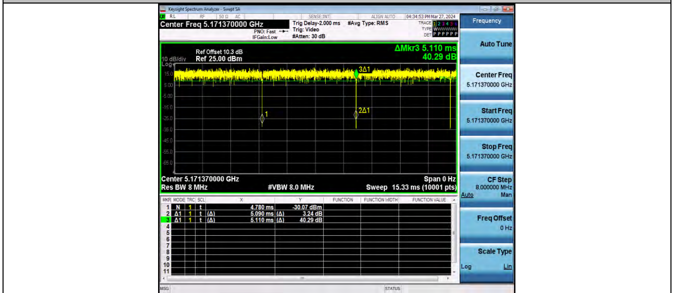
11AX20MIMO_Ant2_5180_52Tone_RU37
