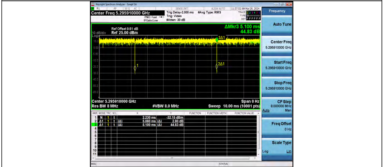
11AX20MIMO_Ant1_5300_106Tone_RU53
