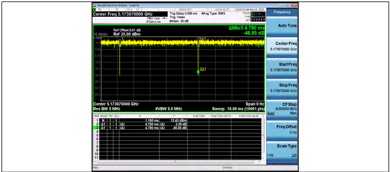
11AX20MIMO_Ant2_5180_26Tone_RU0
