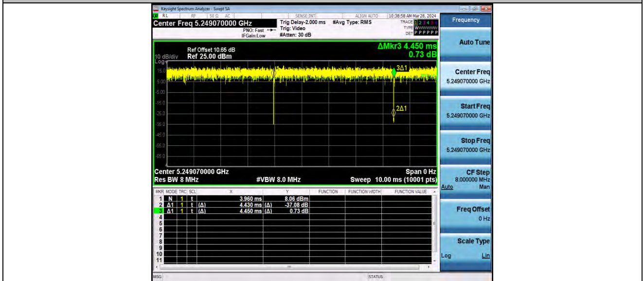
11AX20MIMO_Ant2_5240_52Tone_RU40
