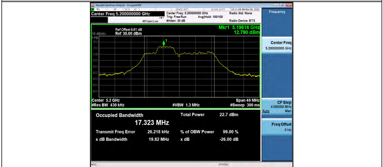
11AX20MIMO_Ant1_5200_106Tone_RU53
