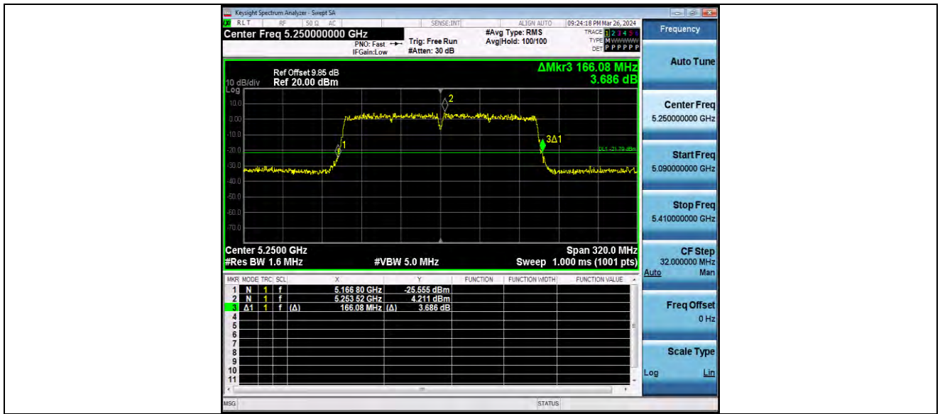
11AC160MIMO_Ant2_5250
