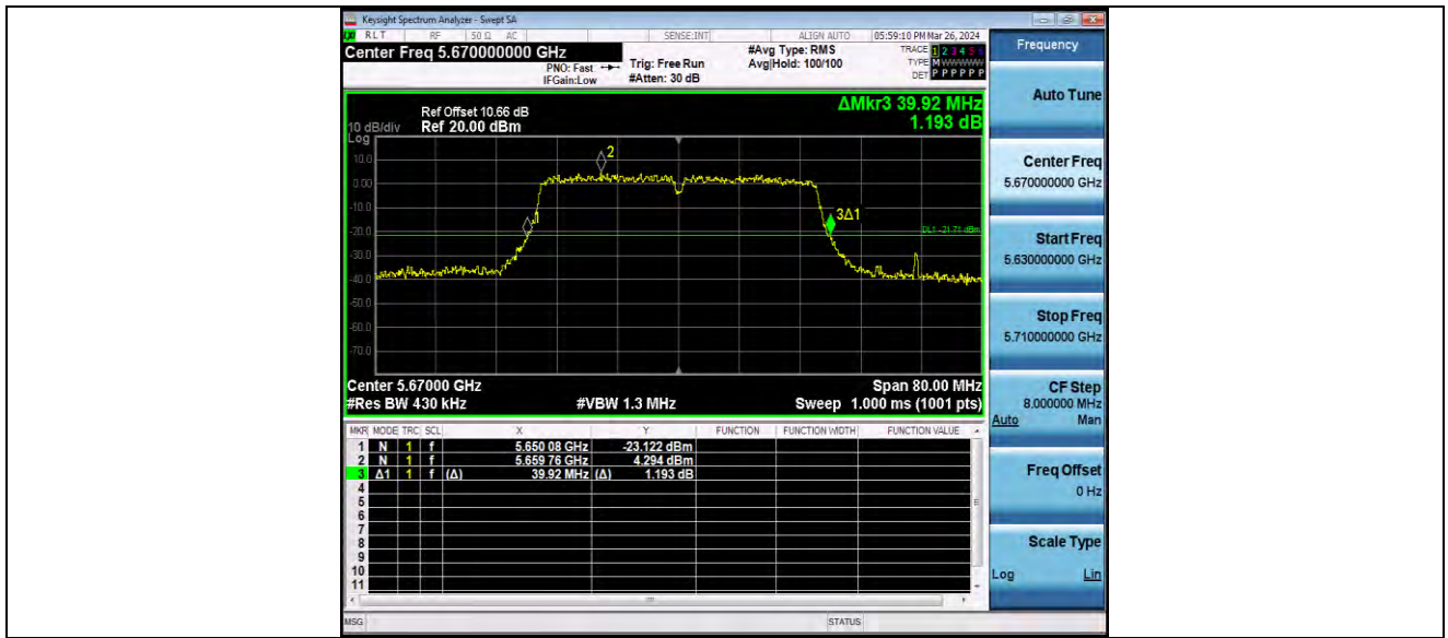
11N40MIMO_Ant2_5670
