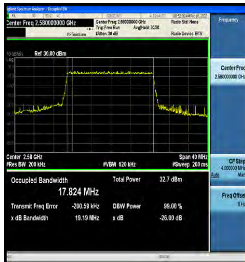
1-N38-30-20-L-2-DFT-PI2BPSK-Outer_Full-50@0-A nt2-17.824-19.19-≤20-PASS
