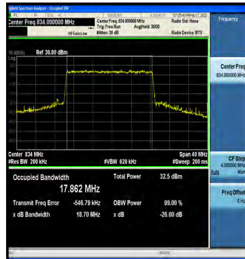
1-N5-15-20-L-1-DFT-QPSK-Outer_Full-100@0-Ant0 17.862-18.70≤20-PASS
