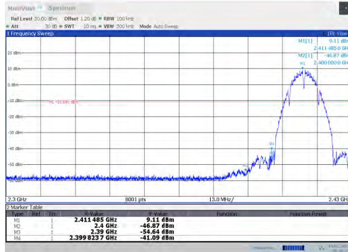
11B-CDD_Ant18_Low_2412
