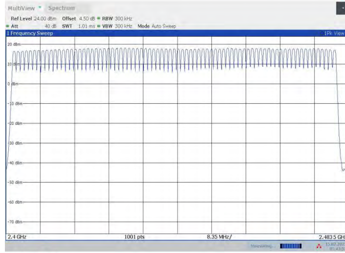
2DH5_Ant16_Hop
