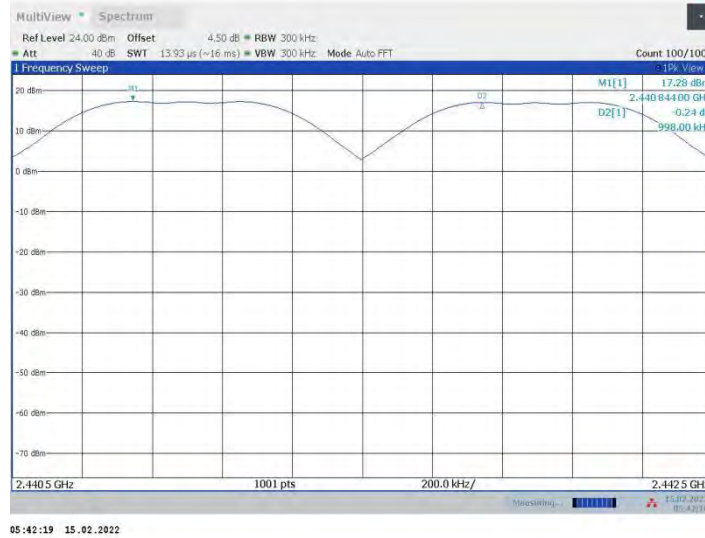
2DH5_Ant16_Hop
