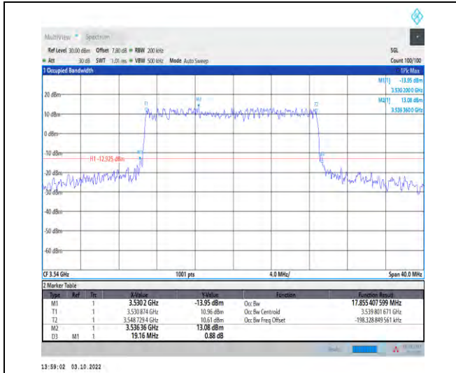
1-N78-3450-3550--30-20-H-3-DFT-16QAM-Outer_Full-50@0-Ant1-17.855-19.160-≤20-PASS
