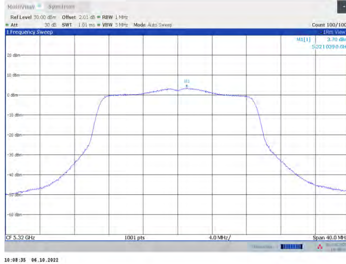
11n20MIMO_Ant8_5320
