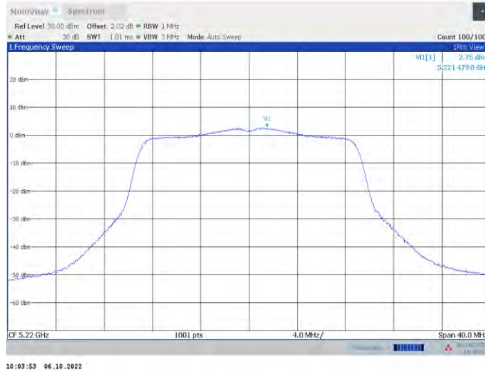
11n20MIMO_Ant8_5220
