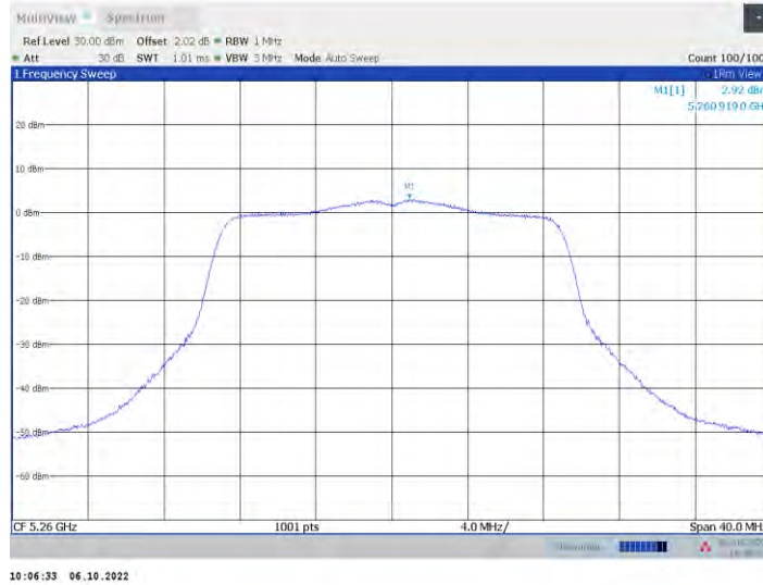
11n20MIMO_Ant8_5260
