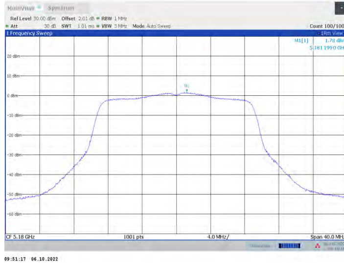
11n20MIMO_Ant8_5180
