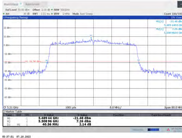
11x40MIMO_Ant8_5510
