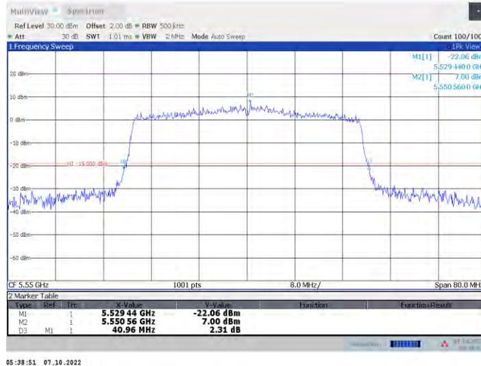
11x40MIMO_Ant8_5550
