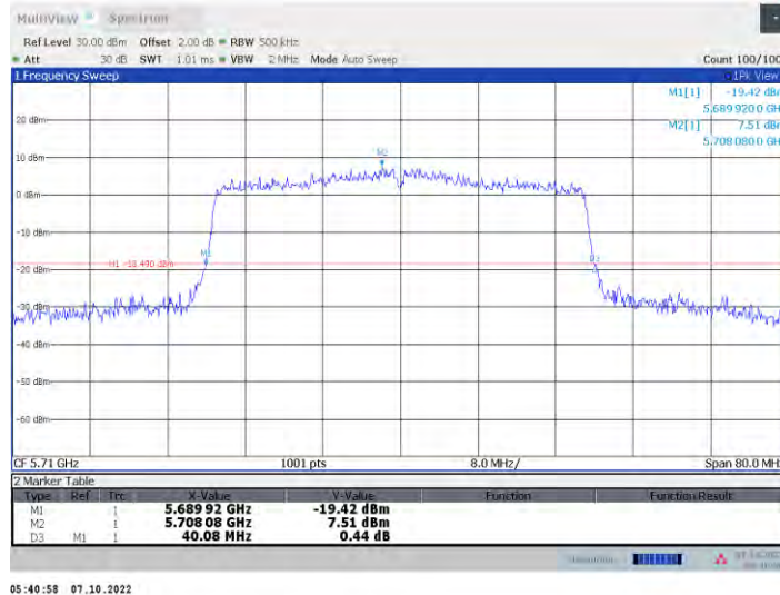
11x40MIMO_Ant8_5710
