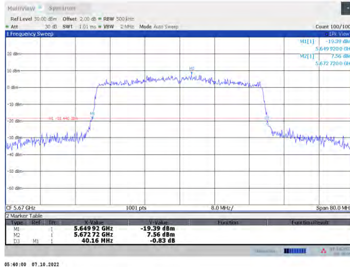
11x40MIMO_Ant8_5670
