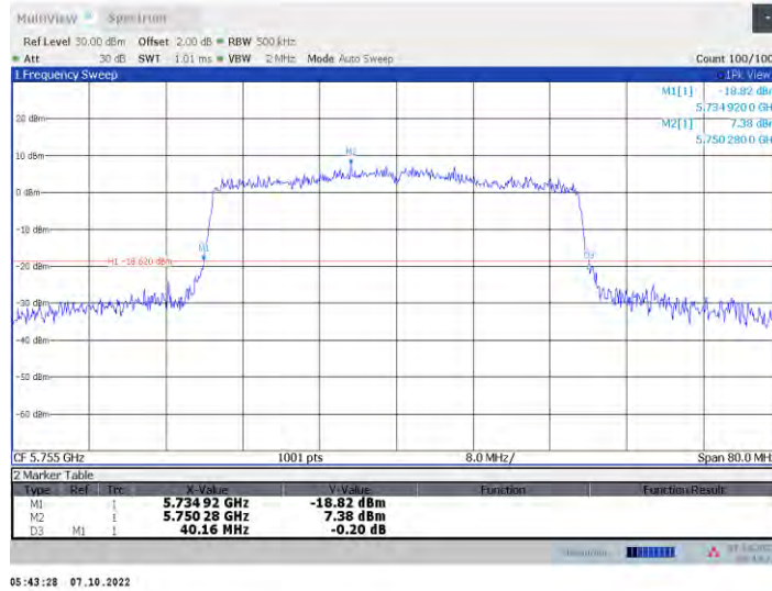
11x40MIMO_Ant8_5755
