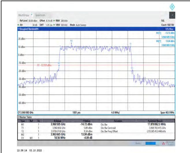
1-N77-3700-3980--30-20-H-3-DFT-16QAM-Outer_Fu II-50@0-Ant1-17.819-18.560-≤20-PASS
