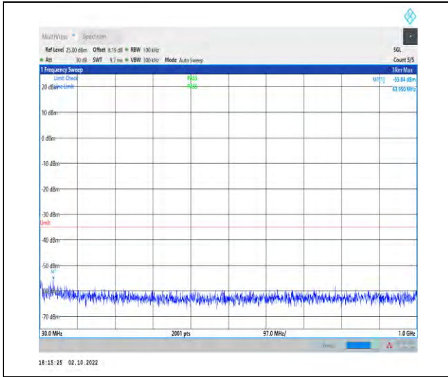
1-N7--15-50-M-1-DFT-PI2BPSK-Inner_1RB_Left-1 @ 1-30-1000-Ant1-63.95--55.84--35-PASS
