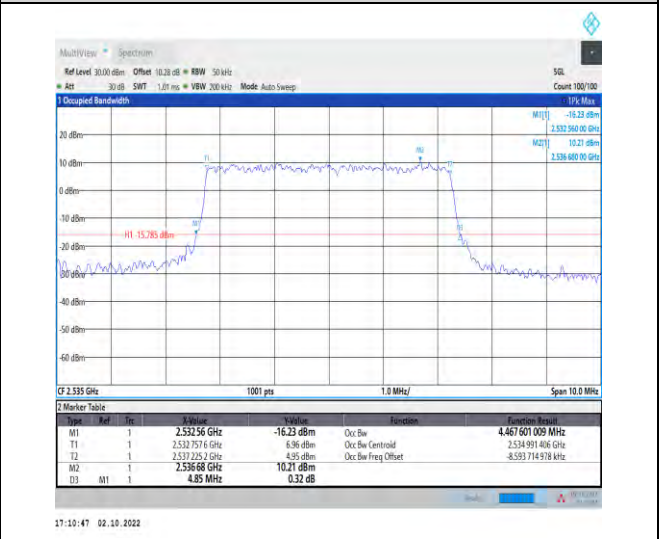
1-N7--15-5-M-7-CP-16QAM-Outer_Full-25@0-Ant1- 4.468-4.850-≤5-PASS
