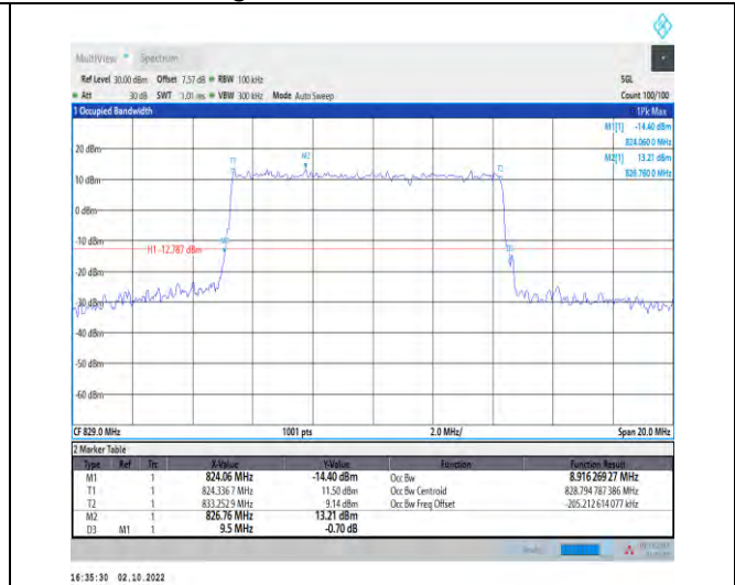
1-N5-PC3-15-10-L-3-DFT-16QAM-Outer_Full-50@0-Ant1-8.916-9.500-≤10-PASS
