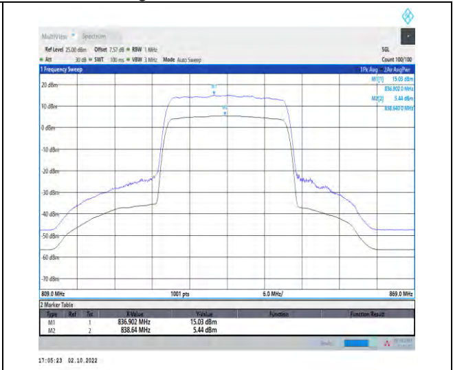
1-N5-PC3-15-20-H-2-CP-256QAM-Outer_Full-106@ 0-Ant1-9.59-100%-0.00-9.59-PASS-≤13
