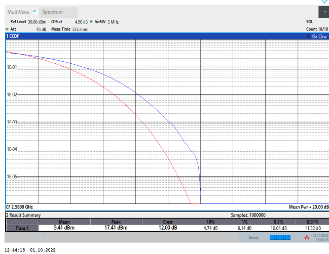
38-38-20MHz-20MHz-QPSK-QPSK-37901-38099-100RB#0-100RB#0
