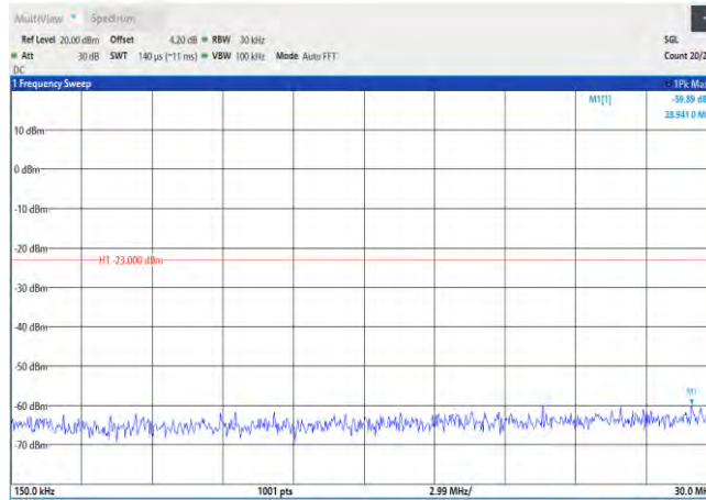
BandII-9262-0.15~30MHz
