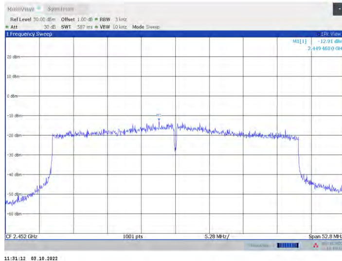
11ax40MIMO_Ant8_2452
