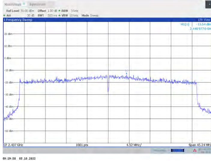
11ax40MIMO_Ant8_2437
