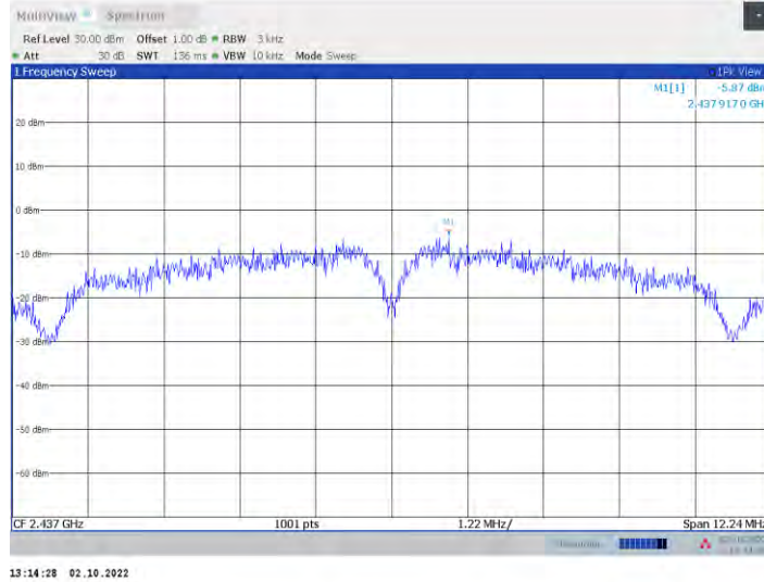
11b-CDD_Ant8_2437
