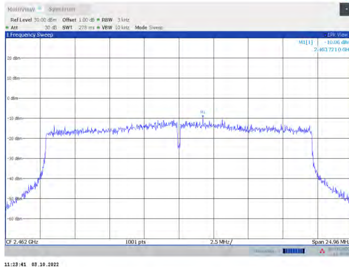
11ax20MIMO_Ant8_2462
