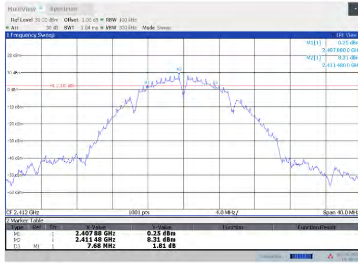
11b-CDD_Ant8_2412
