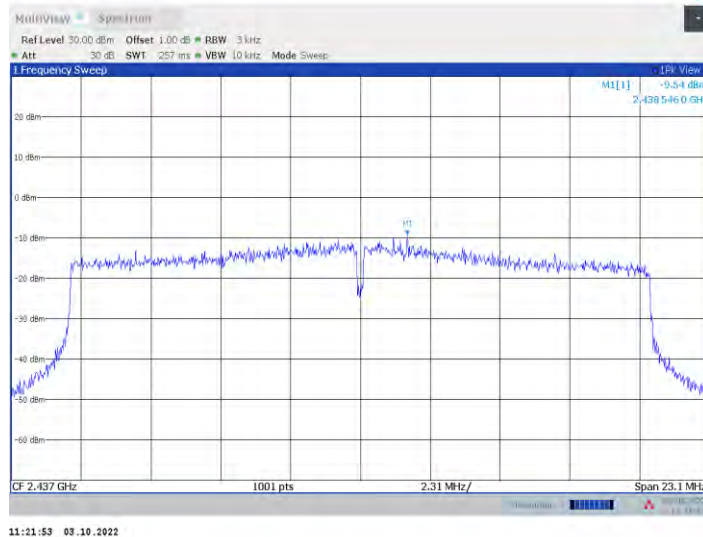
11ax20MIMO_Ant8_2437
