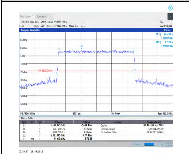
1-N78-3700-3800--30-90-L-9-CP-256QAM-Outer_Fu II-245@0-Ant1-87.433-91.080-≤90-PASS
