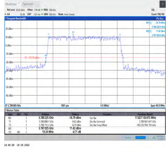
1-N78-3700-3800--30-20-H-4-DFT-64QAM-Outer_Fu II-50@0-Ant1-17.827-19.240-<20-PASS
