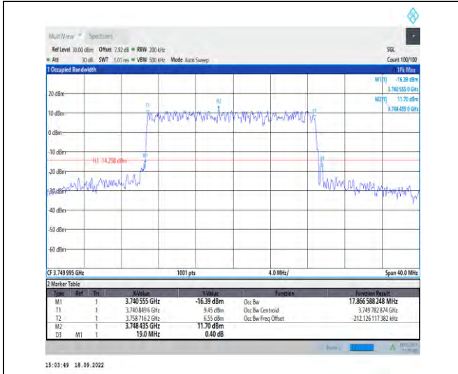
1-N78-3700-3800--30-20-M-4-DFT-64QAM-Outer_Full-50@0-Ant1-17.867-19.000-≤20-PASS
