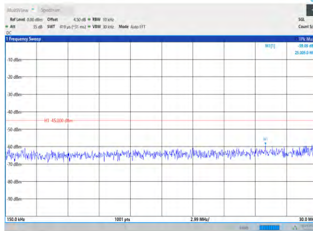
Band38-20MHz-QPSK-37850-1RB#0-Range2:0.15~30MHz
