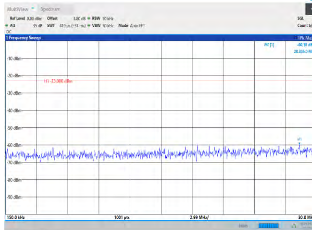
Band12-10MHz-QPSK-23060-1RB#0-Range2:0.15~30MHz
