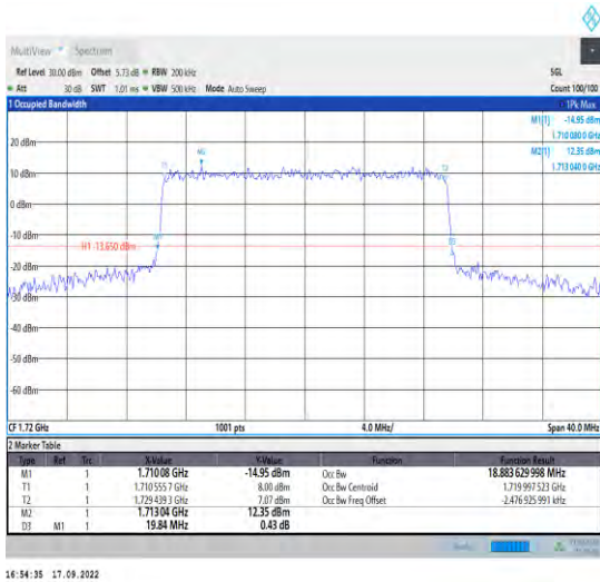
1-N66--15-20-L-6-CP-QPSK-Outer_Full-106@0-Ant1 -18.884-19.840-≤20-PASS
