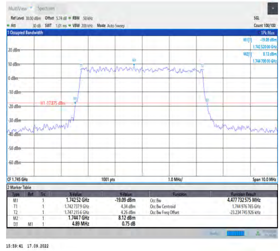
1-N66--15-5-M-9-CP-256QAM-Outer_Full-25@0-Ant 1-4.478-4.890-≤5-PASS
