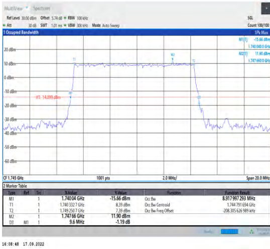
1-N66--15-10-M-5-DFT-256QAM-Outer_Full-50@0-A nt1-8.918-9.600-≤10-PASS
