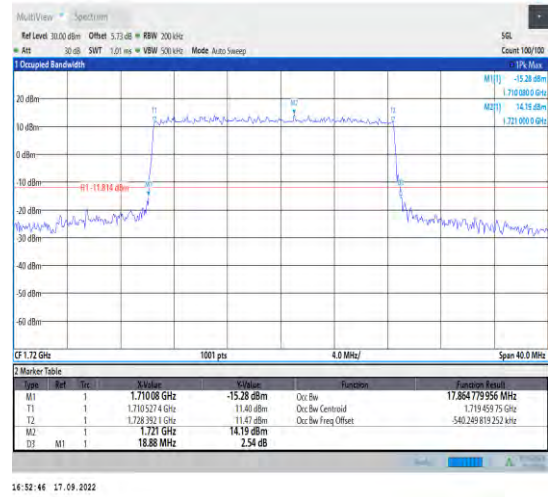
1-N66--15-20-L-1-DFT-QPSK-Outer_Full-100@0-Ant 1-17.865-18.880-≤20-PASS
