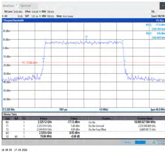
1-N7--15-20-M-9-CP-256QAM-Outer_Full-106@0-A nt1-18.905-19.840-≤20-PASS
