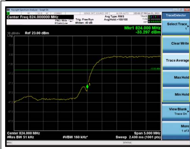
LTE Band 5 QPSK 1.4MHz CH-Low 1RB
