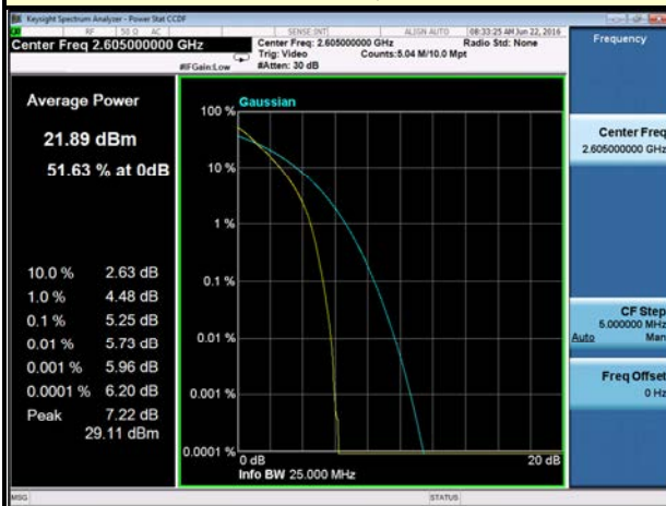
20MHz / QPSK
