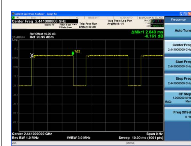
Modulation: \pi/4 DQPSK 2DH5 2441
