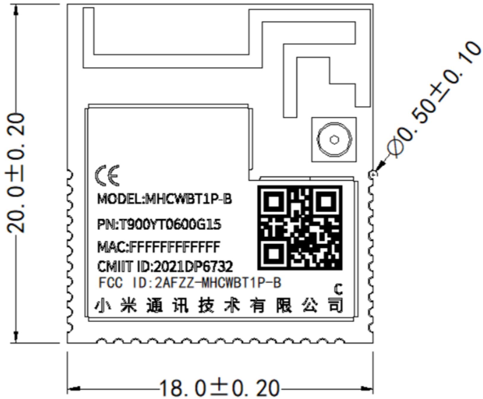
主视图
