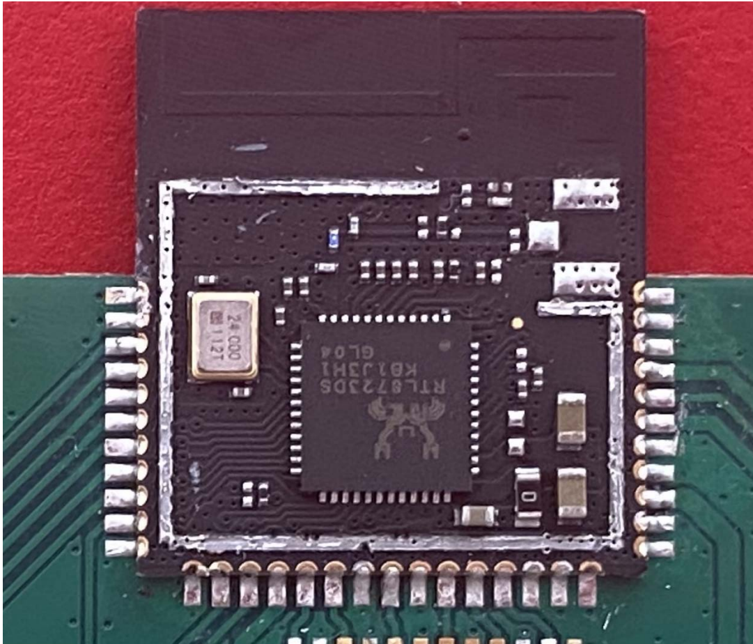
IC Details 2
