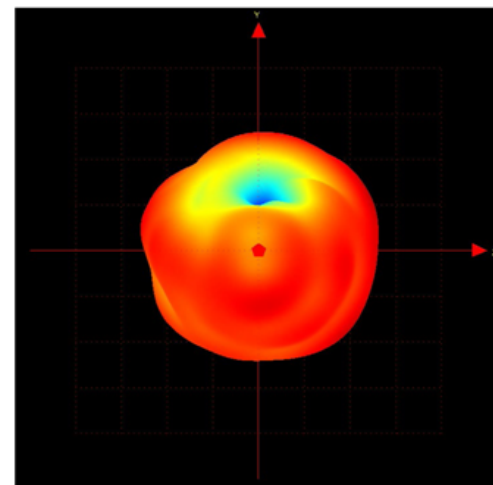
Z 2440MHz
