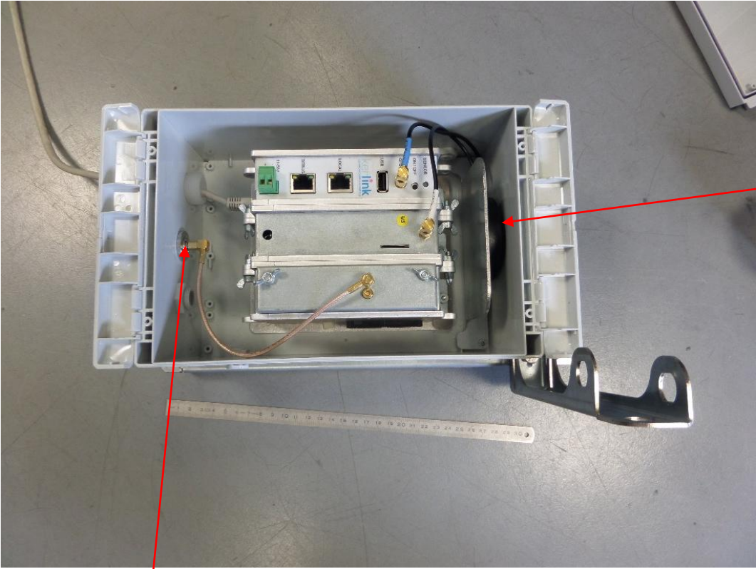
GPS/LTE antenna
