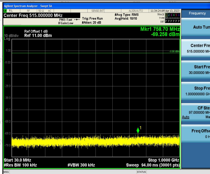
2.4G_Ant1_2436_30~1000
