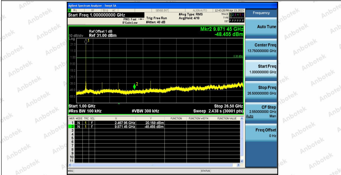
2.4G_Ant1_2468_1000~26500
