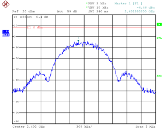
Test Mode : ANT1 Low channel
