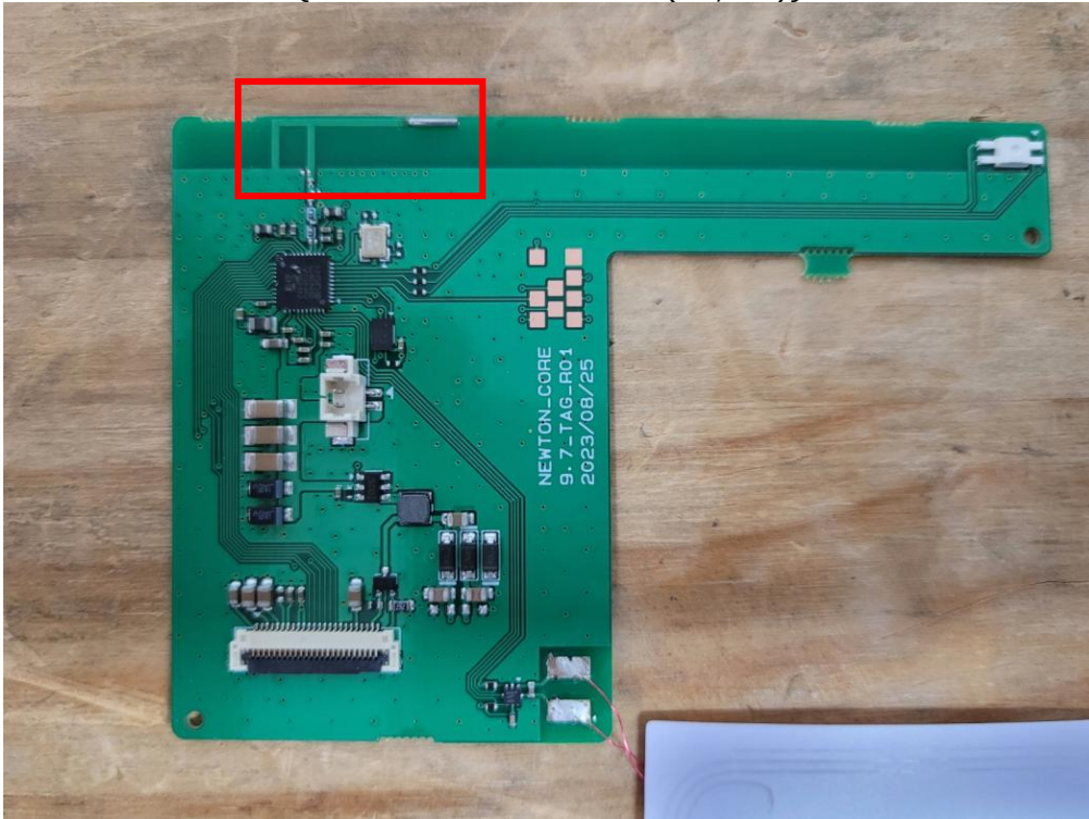
{NFC Antenna(RX)}
