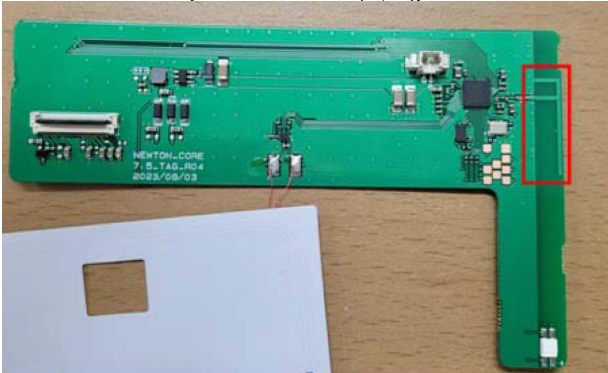
{NFC Antenna (RX)}
