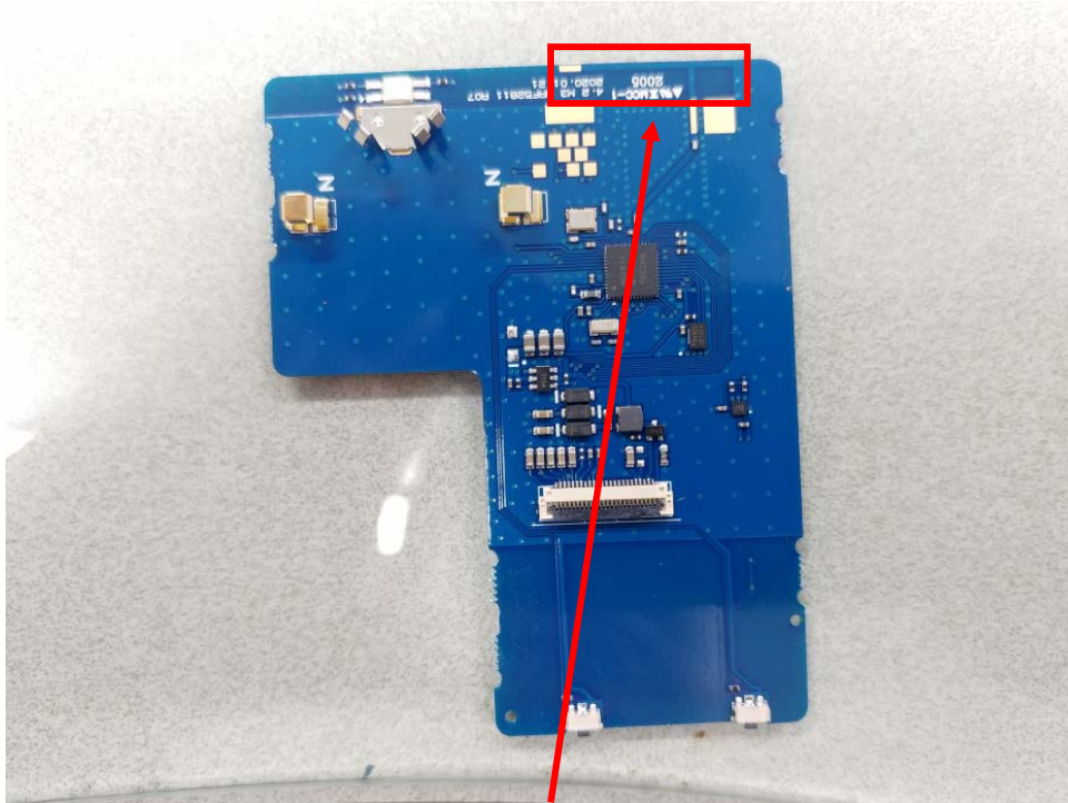
Antenna(TX, RX)
