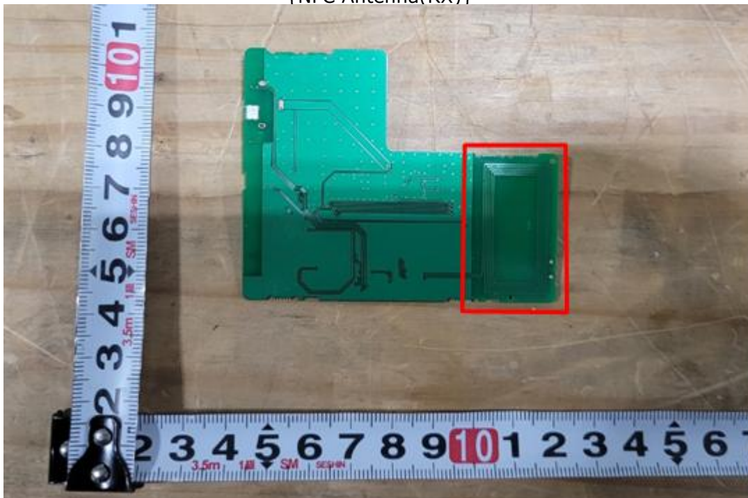
{NFC Antenna(RX)}
