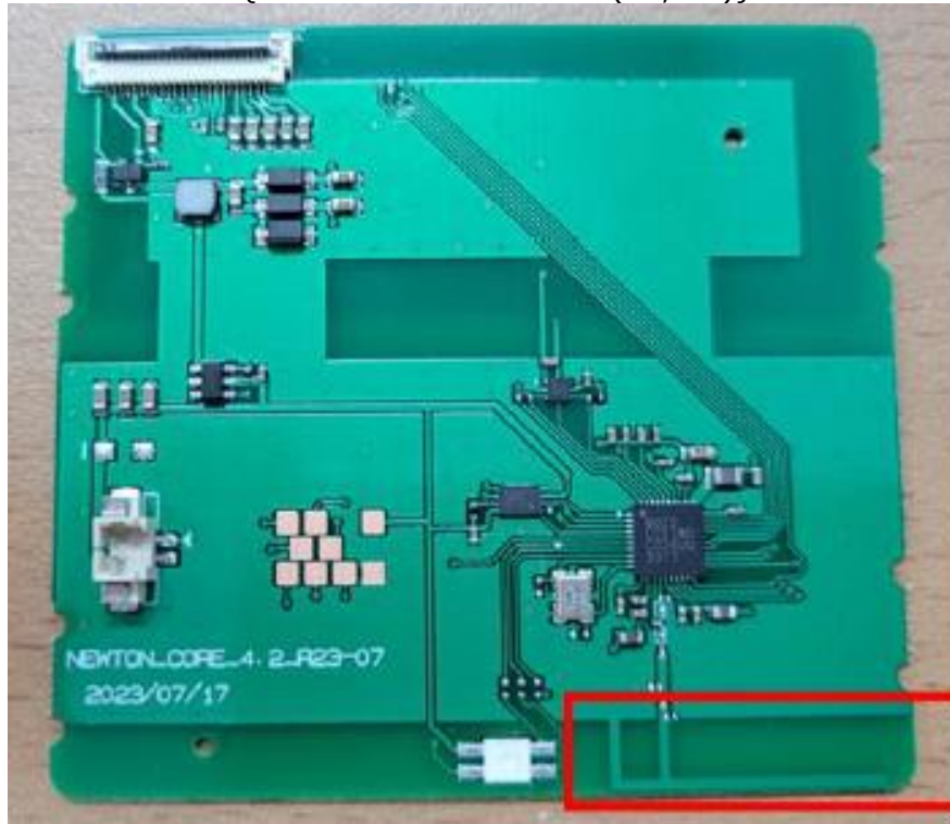
{NFC Antenna (RX)}
