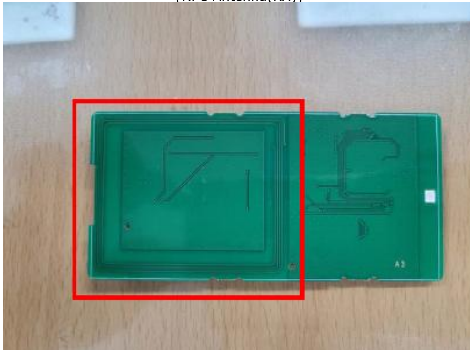
{NFC Antenna(RX)}
