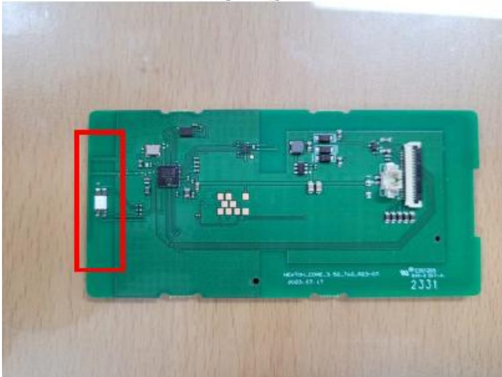
{NFC Antenna(RX)}
