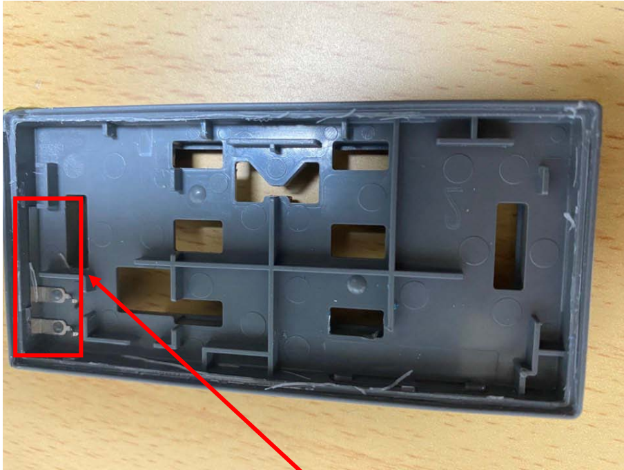
Antenna(TX, RX)
