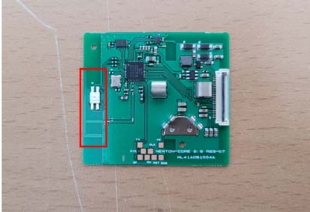
{ NFC Antenna (RX)}
