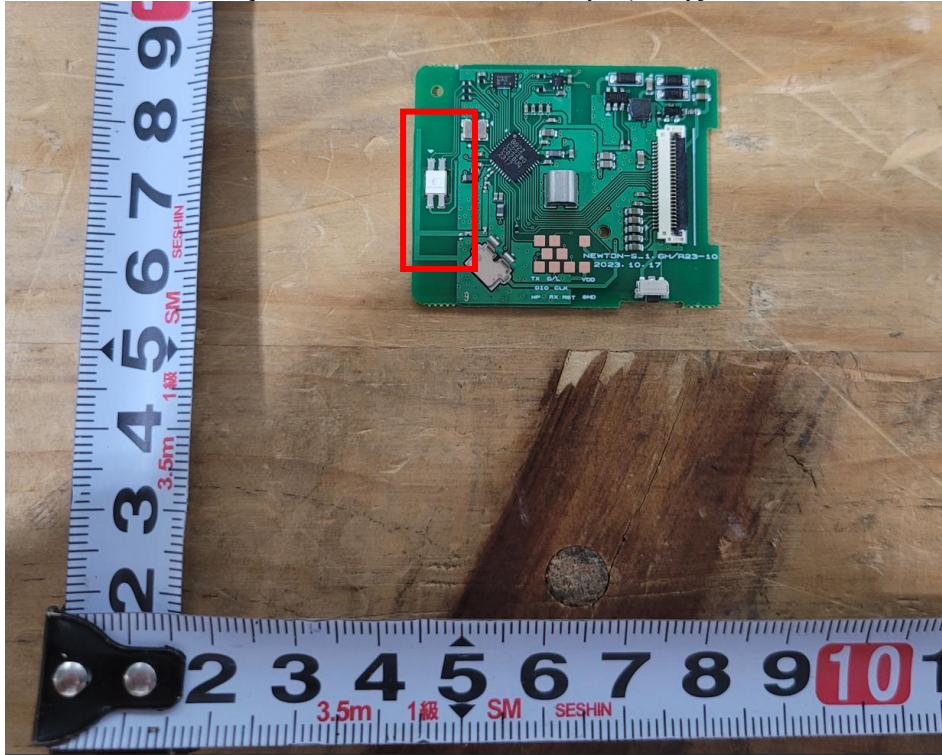
{NFC Antenna(RX)}
