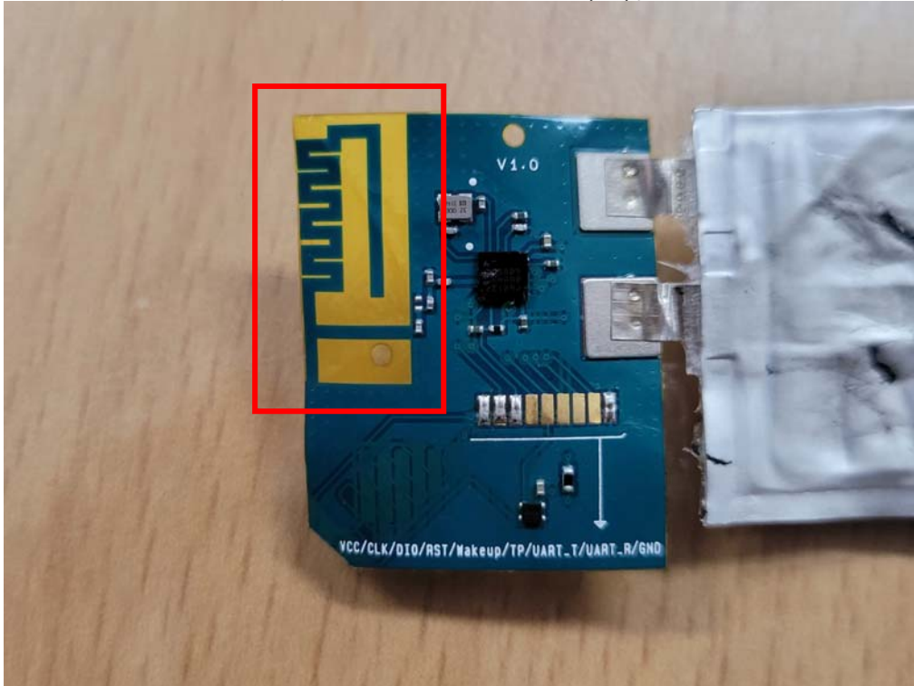
{ 2402-2480MHz Antenna(TX) }
