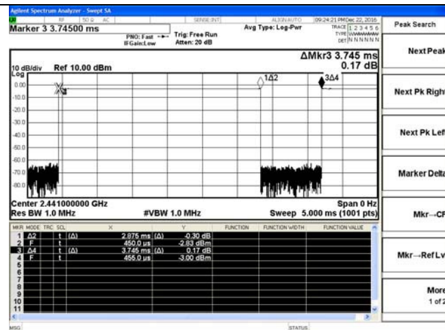
DH5-2441MHz)
