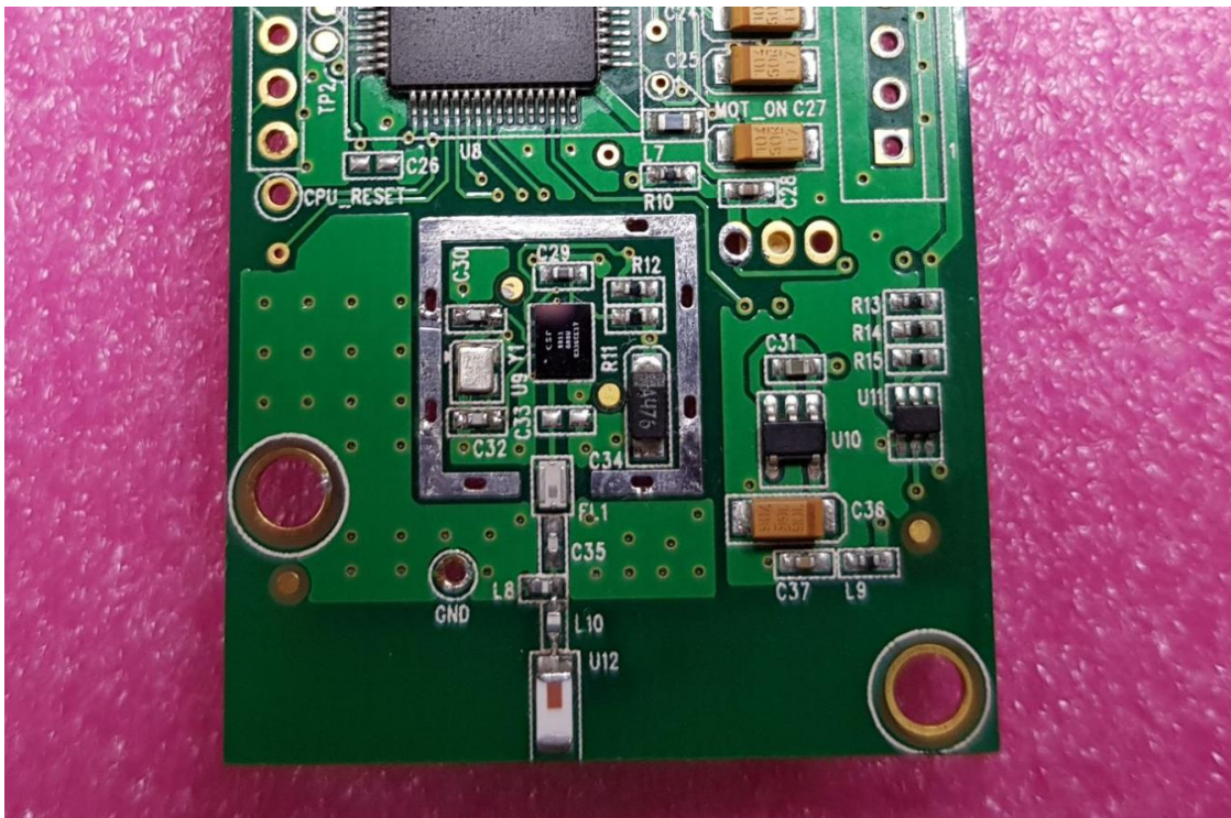
EUT RF Module without shield
