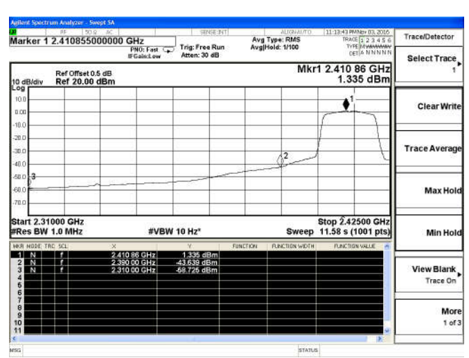
802.11n(HT20)-Low channel(Average)
