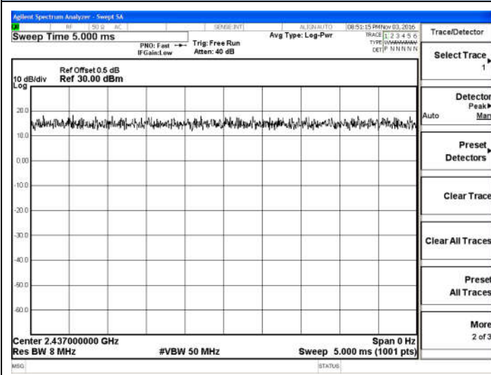
802.11n-HT20
