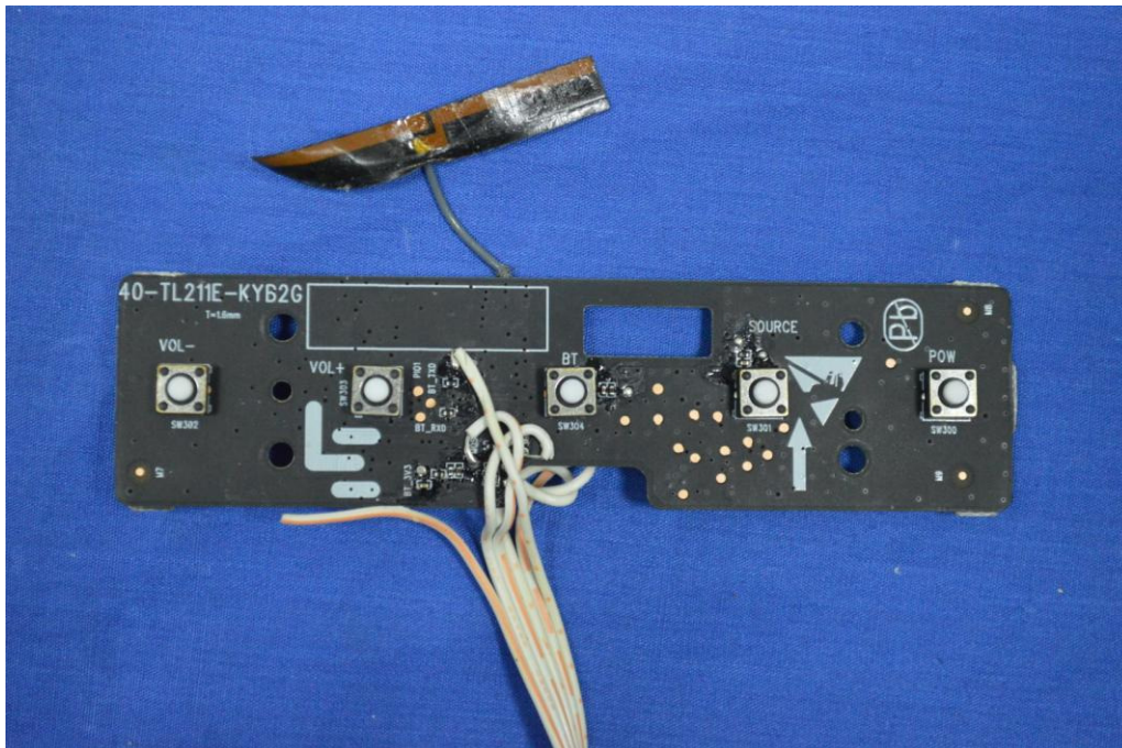
(10) EUT Photo
