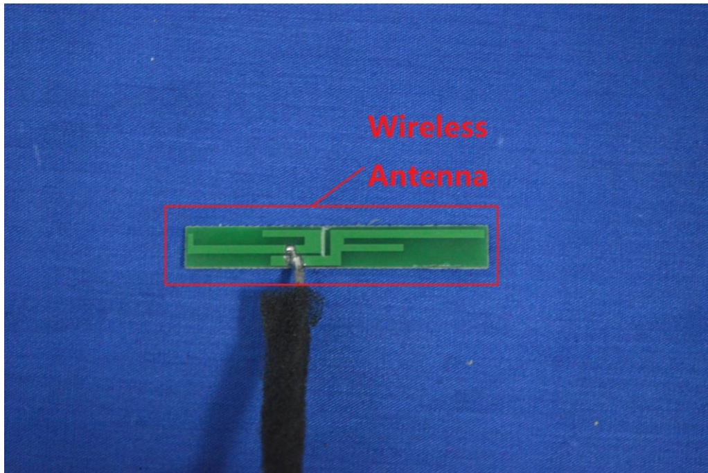
(8) EUT Photo
